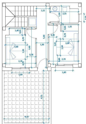
PLANTA PRIMERA
