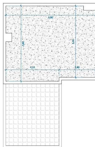
CUBIERTA
