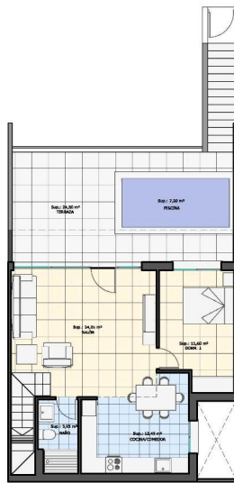
PLANTA BAJA
